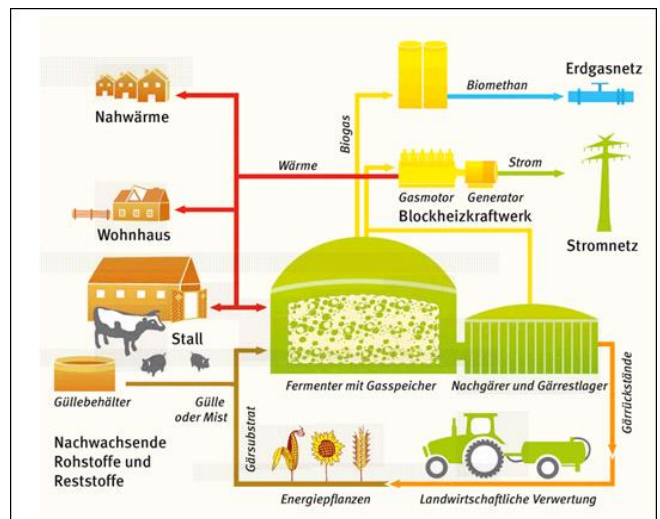
Schema Nahwärmenetz
